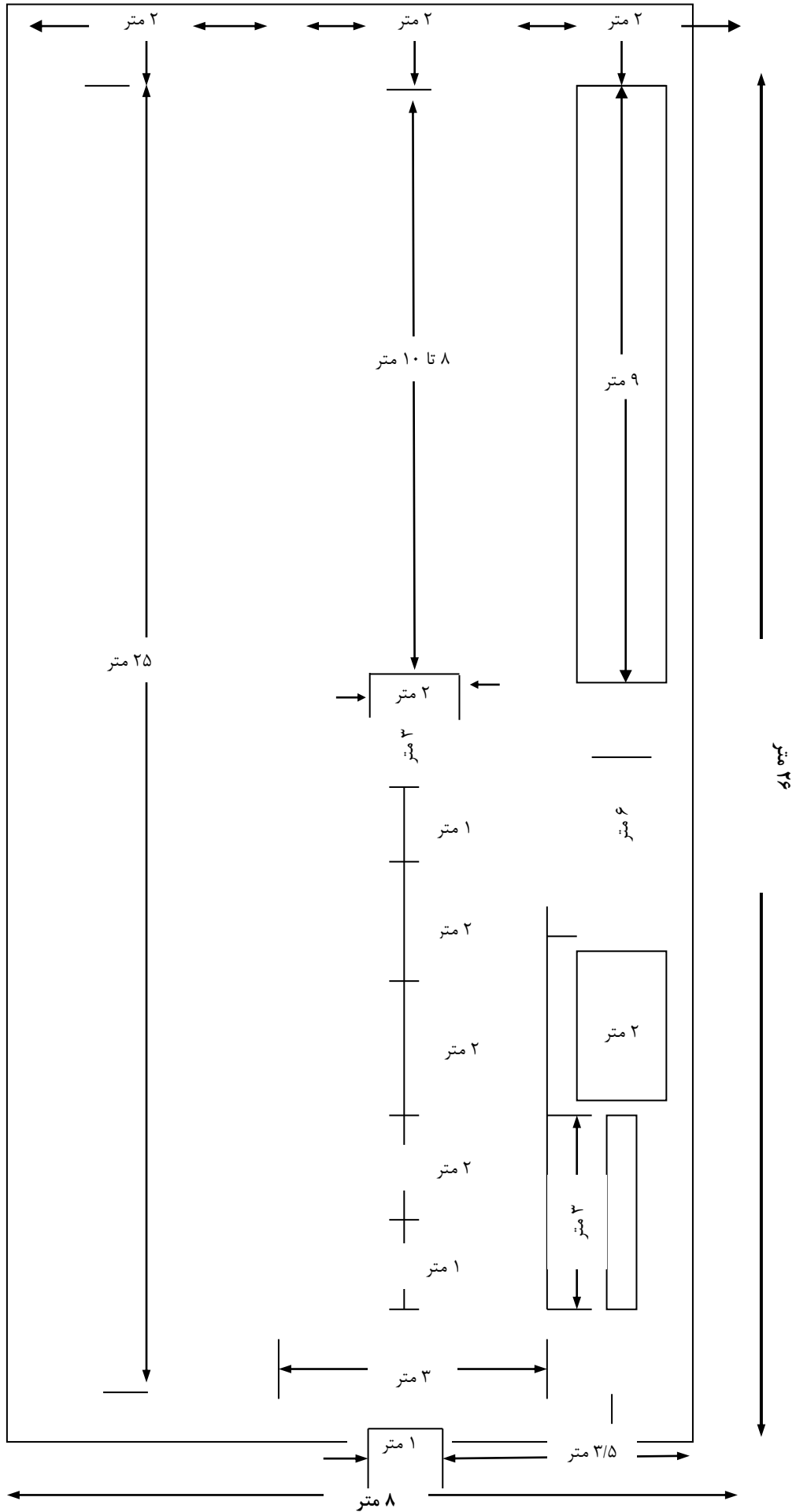
شکل ۳- جانمایی نقشه ایستگاه‌های آزمون عملی در یک مجموعه آزمون
